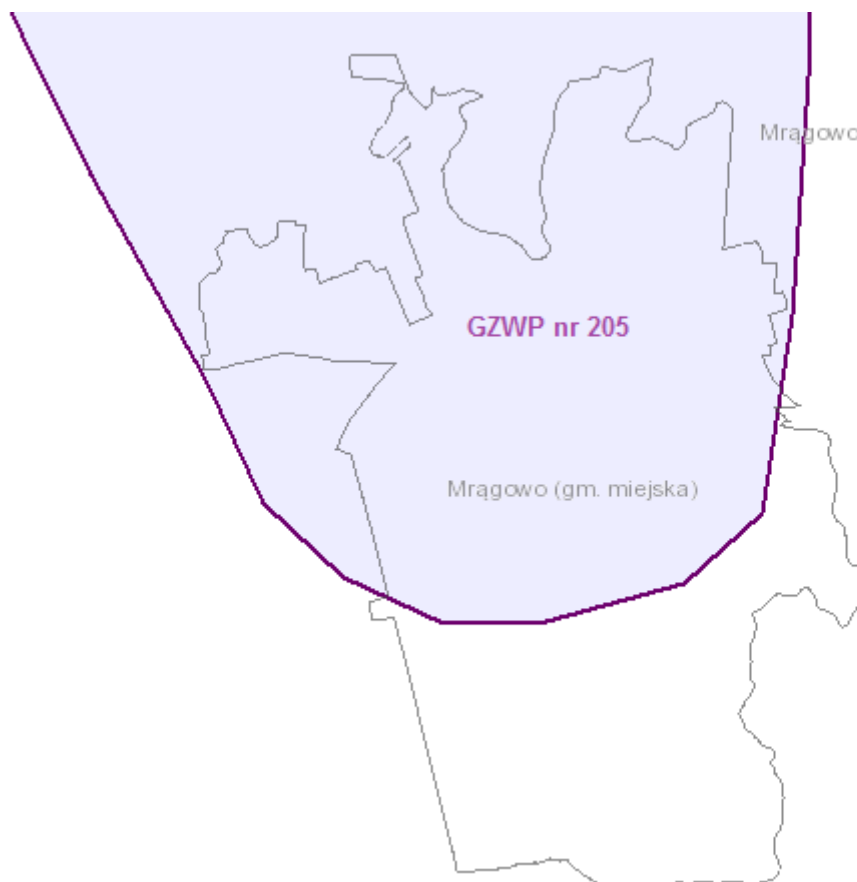
Rysunek 6. Miasto Mrągowo na tle Głównego Zbiornika Wód Podziemnych nr 205
