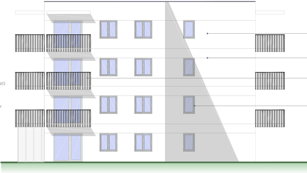
ELEWACJA SZCZYTOWA- PÓŁNOCNA
