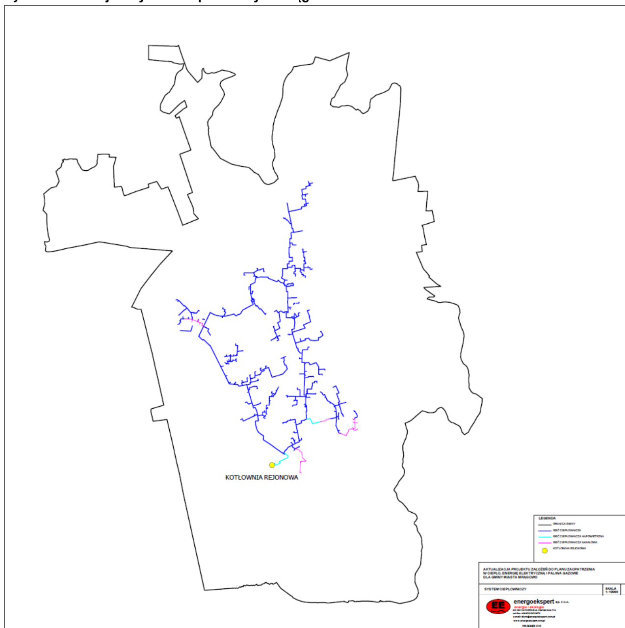
Rysunek 3-2 Miejski system ciepłowniczy w Mrągowie
