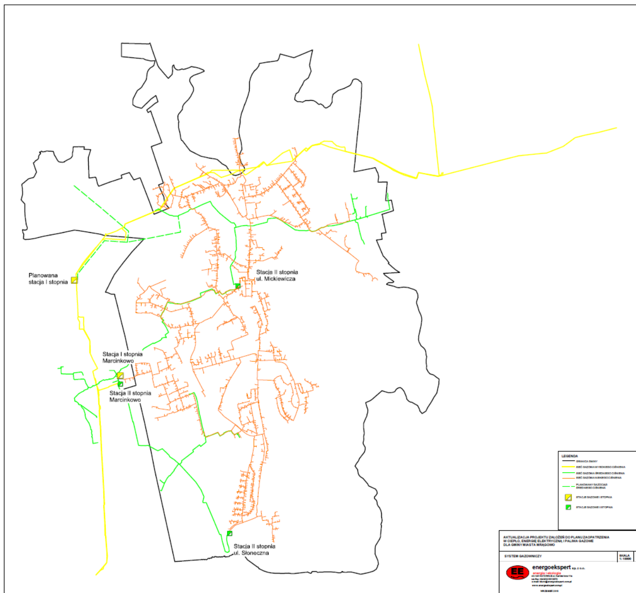
Rysunek 3-5 System dystrybucyjny gazu ziemnego na obszarze miasta Mrągowa
